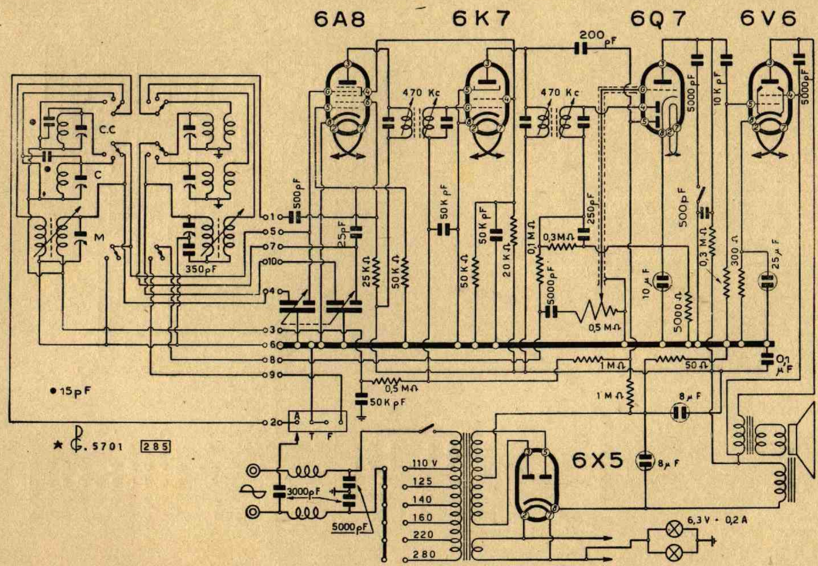
Lo schema elettrico del mod. 653
